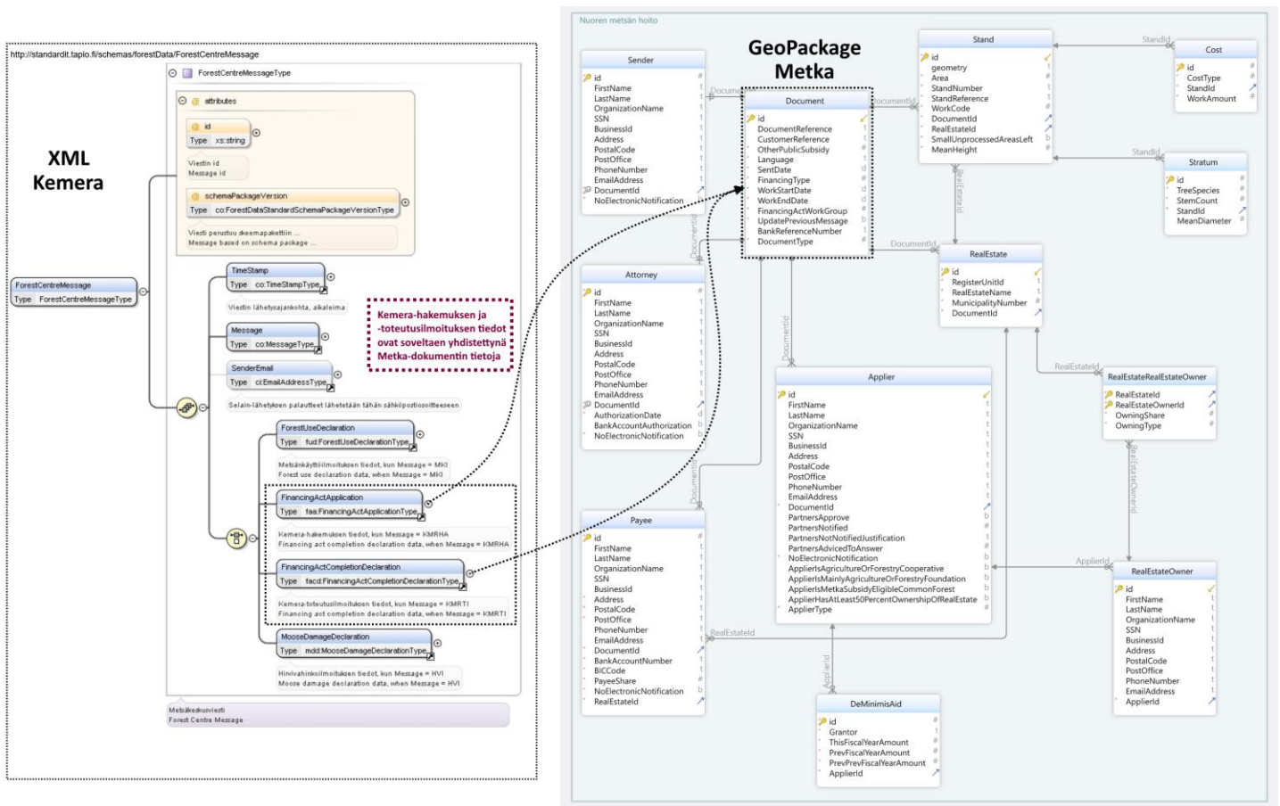
Kuva. Vasemmalla valkoisella pohjalla XML-muotoisen Kemeran tietorakenteita ja oikealla tummimmalla pohjalla GeoPackage-muotoisen Metkan tietorakenteet. Kemera-XML:n juurielementti ForestCentreMessage ja sen alla Kemera-hakemuksen (<FinancingActApplication>) tai -toteutusilmoituksen (<FinancingActCompletionDeclaration>) tiedot. Metkan GeoPackagen keskiössä on Dokumentti (Document) -taulu.
